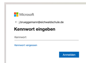
Abbildung 23: Kennworteingabe
